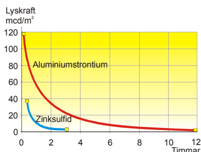
Grafen visar skillnad i lyseffekt mellan efterlysande kristall av zinksulfid och aluminiumstrontium
